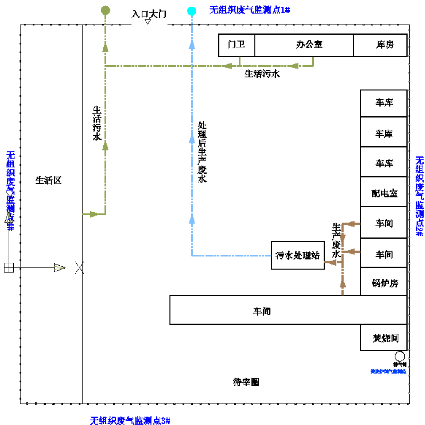
监测点位图
